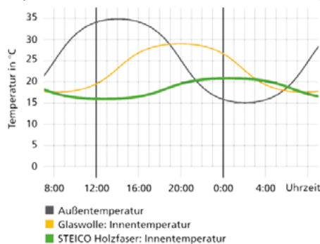
Temperaturverlauf am Dach bei unterschiedlicher Dämmung
