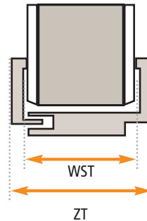
ZT: komplette Tiefe der Zarge WST: Wandstärke einschließlich Putz, Kacheln etc.
