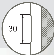
Prägung für Berlin 01 und 03 in Millimetern
