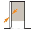
WST: Wandstärke einschließlich Putz, Kacheln etc.
