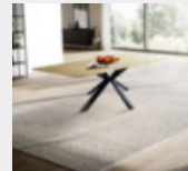
Jupiter
