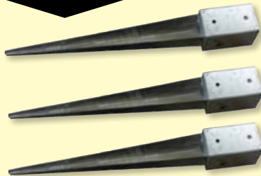
Einschlag- bodenhülle Topflänge 150 mm, 71 x 71 x 750 mm, feuerverzinkt
